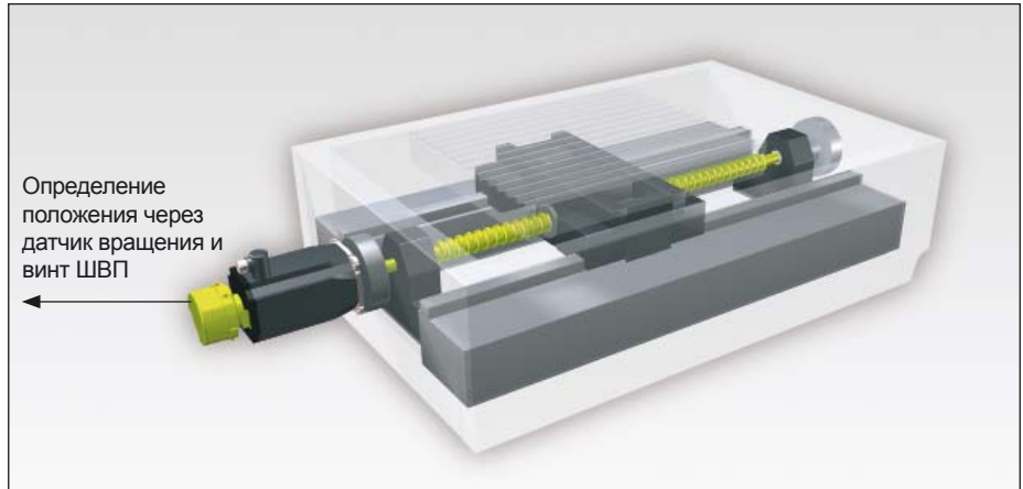
Рисунок 2 Позиционирование в полузамкнутом контуре через ШВП и датчик вращения
