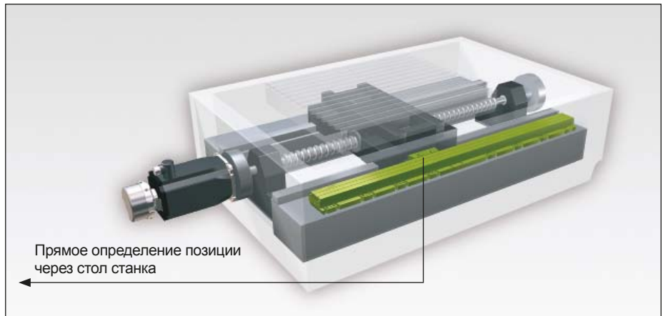
Рисунок 3 Позиционирование в замкнутом контуре при помощи датчика линейного перемещения
