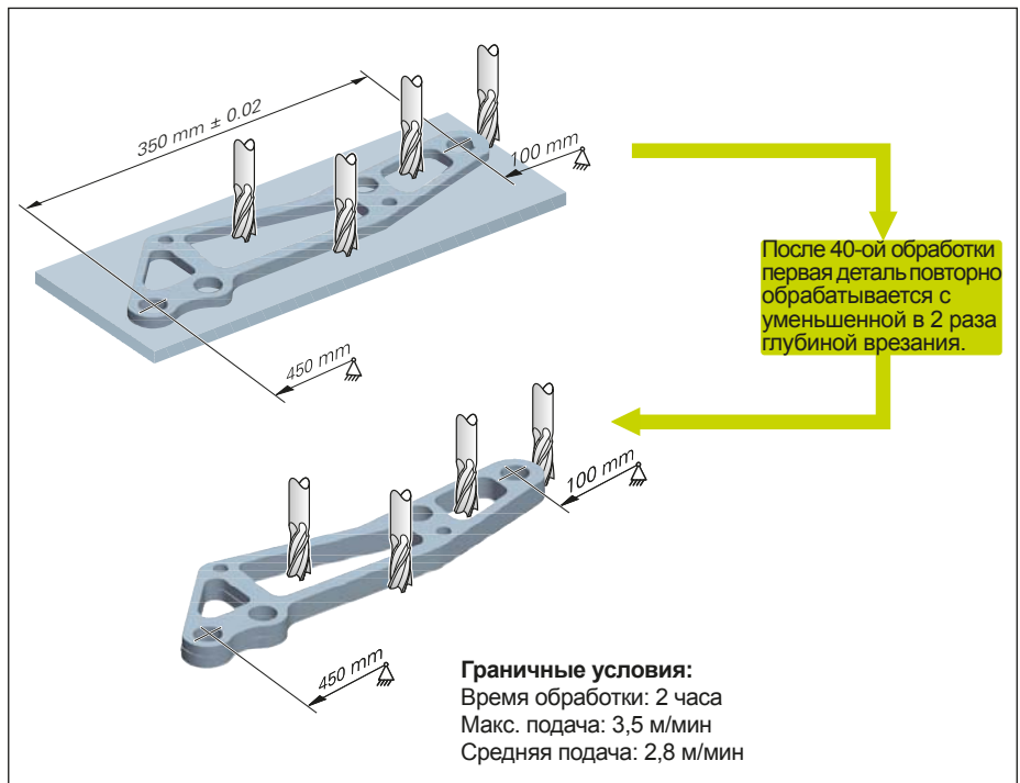
Рисунок 4 Изготовление шарнирного рычага \triangle = точка жесткого крепления опоры ШВП
