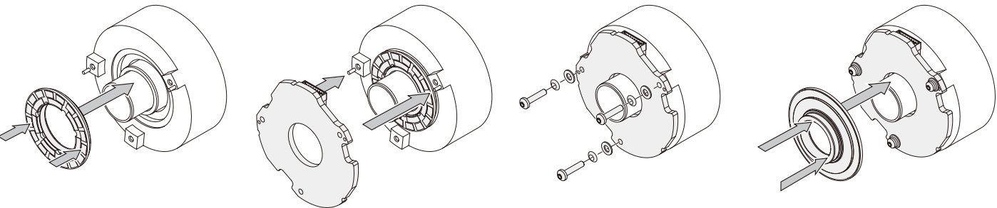
压配的码盘/轴毂组件
