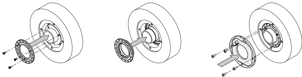
KCI/KBI 1300安装示例
